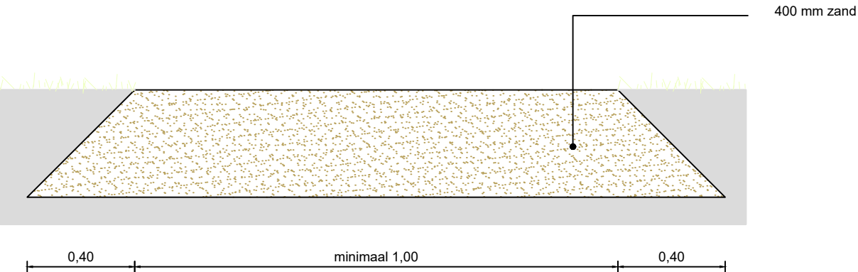
Ruiterpad Schaal 1:20
