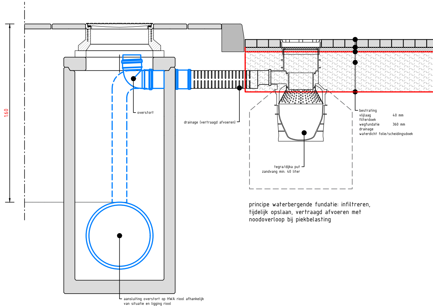
Detail waterbergende bestrating doorsnede Schaal 1:20
