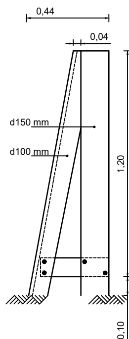
Klaphek zijaanzicht Schaal 1:20
