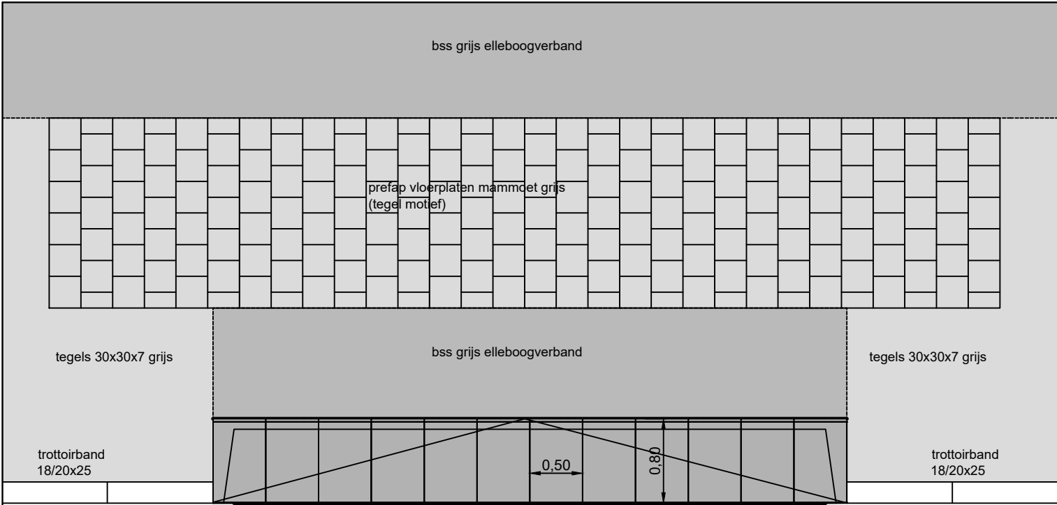
Detail A: inritconstructie Schaal 1:50
