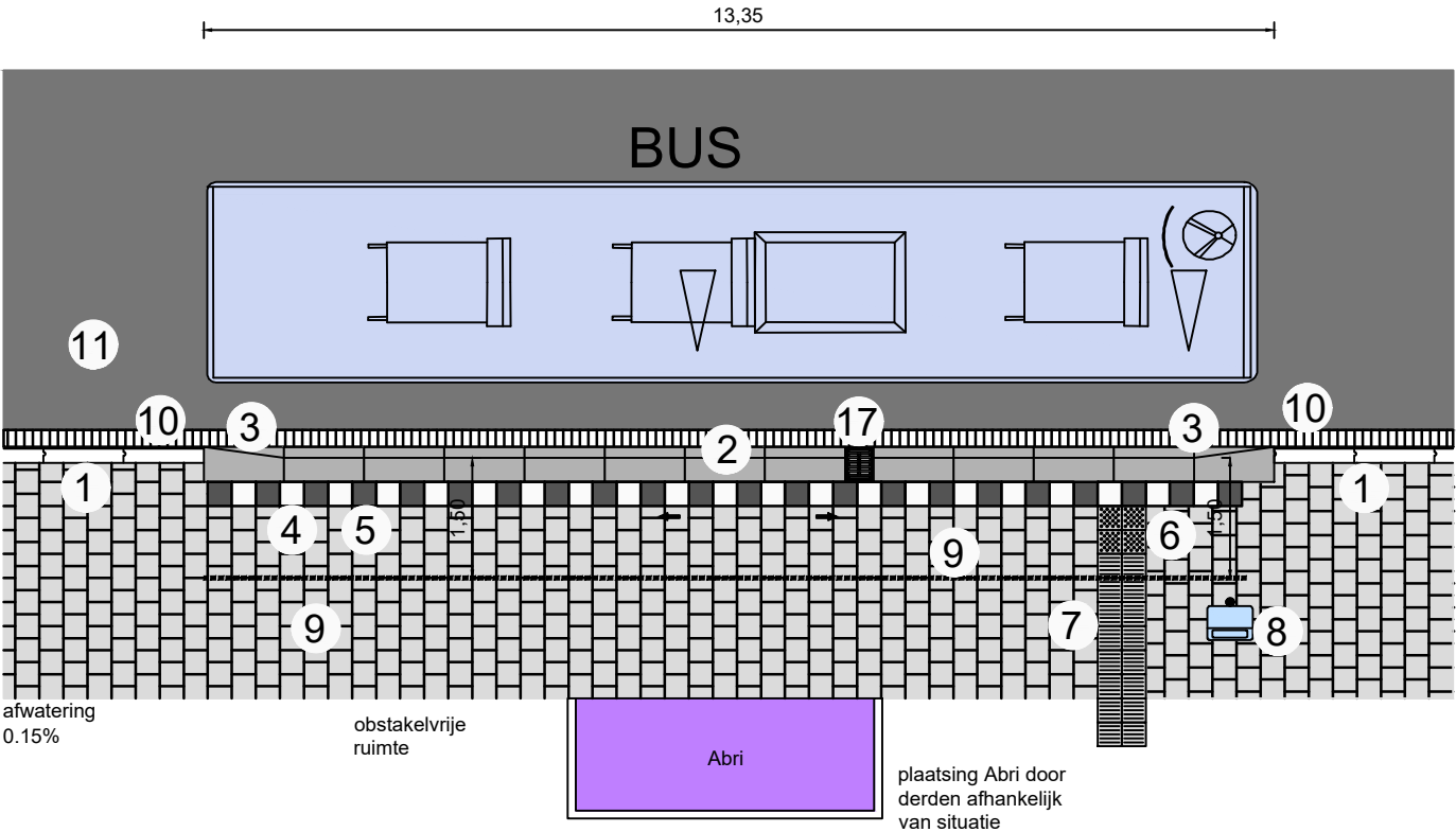
Bushalte 13,35 meter Schaal 1:100
