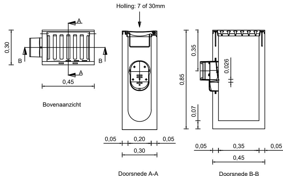
Straatkolk STR-9737 TBS Soest Schaal 1:20
