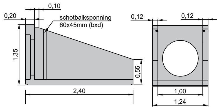
HWA / Drainage Schaal 1:50
