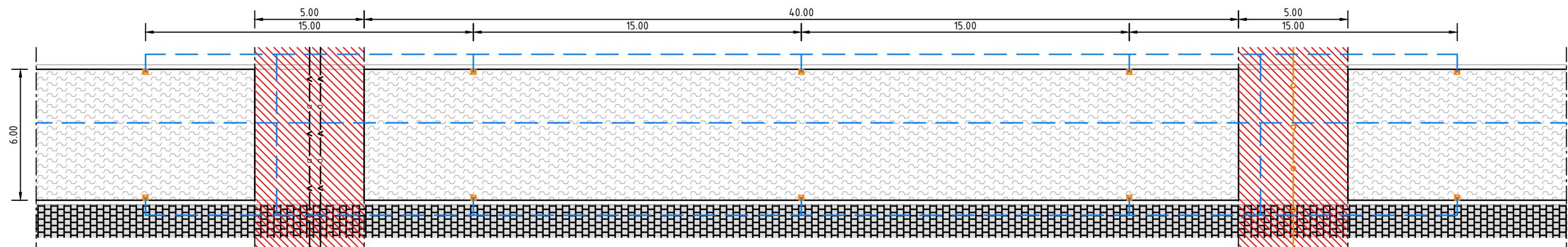
Detail waterbergende bestrating plattegrond Schaal 1:200
