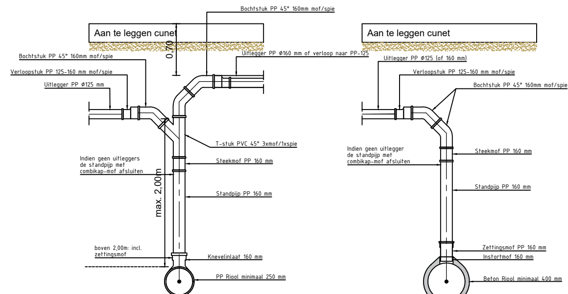
HWA huisaansluiting Schaal 1:50
