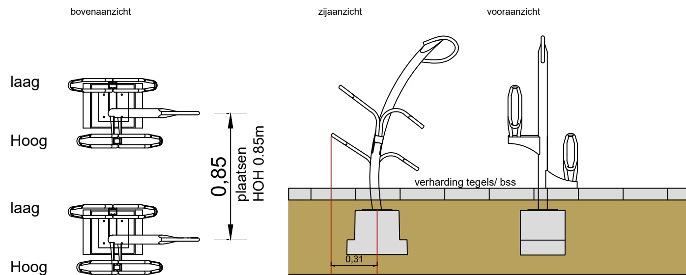
Fietsparkeren Tulip
