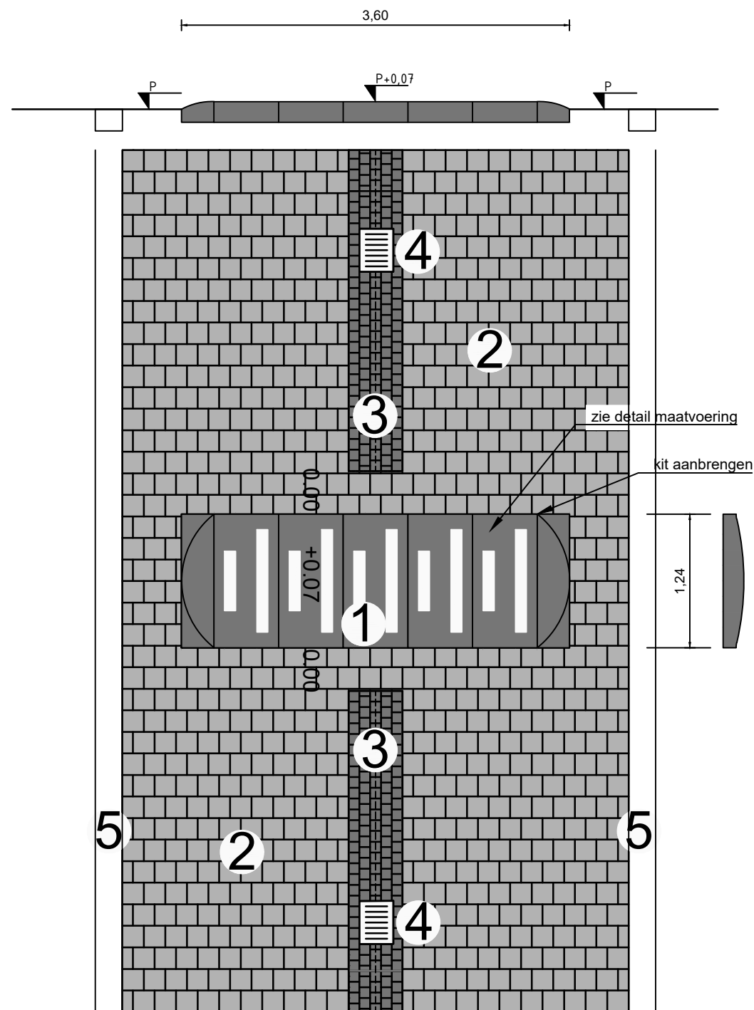
Principe detail: kussendrempel beton schaal 1:50
