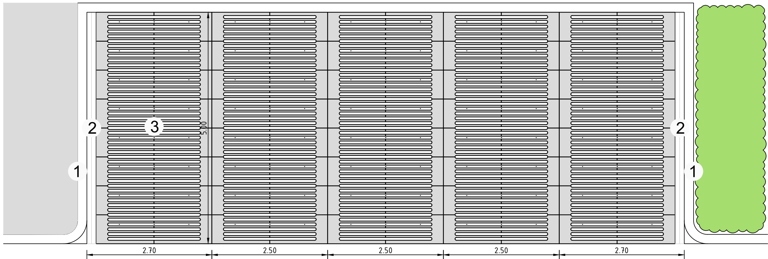
Principe detail: haaksparkeren grasbetontegels 1:50
