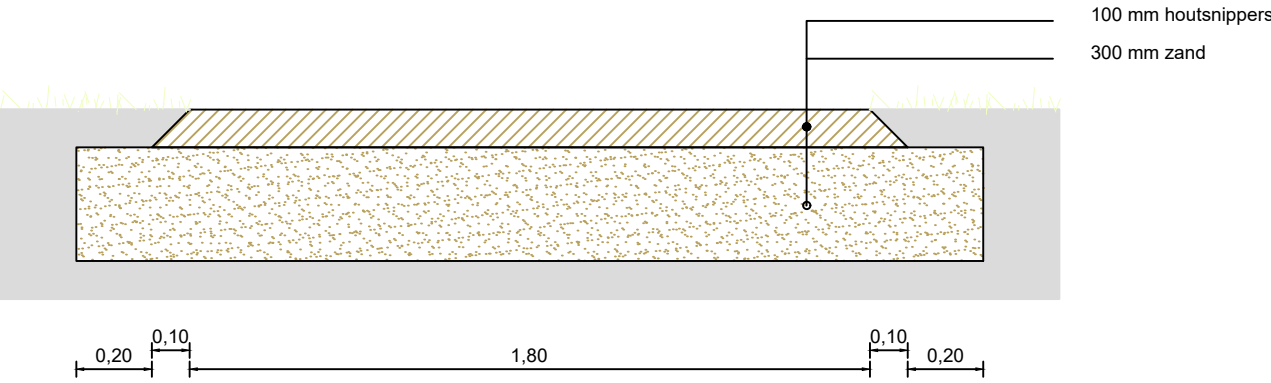
Voetpad met houtsnippers Schaal 1:20
