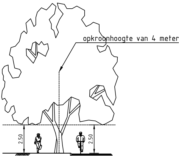
Profiel van vrije ruimte bij fietspad, trottoir en parkeervak Schaal 1:200
