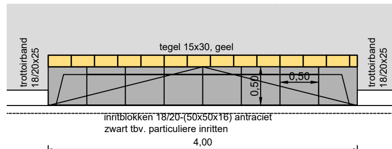
Detail C: inritconstructie Schaal 1:50
