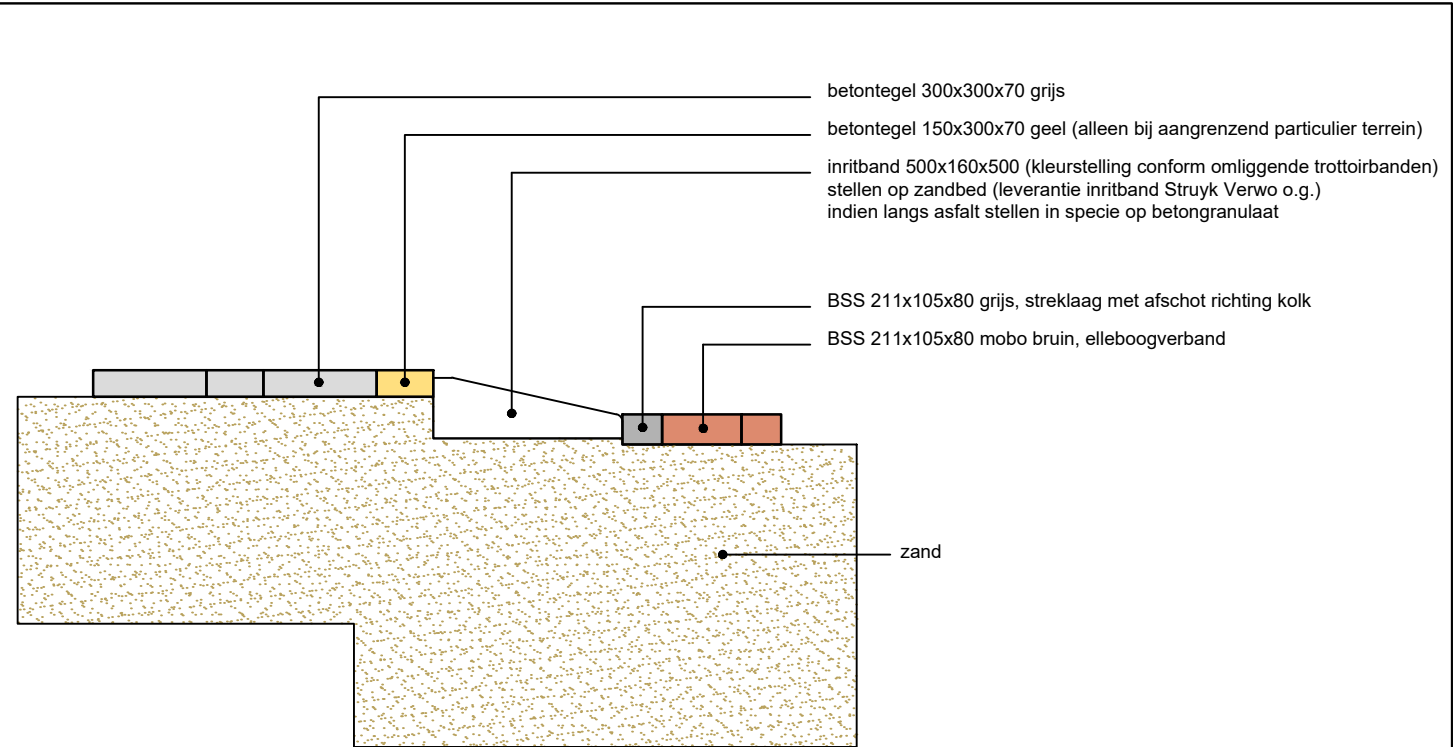
Inritblok 50x16x50 (inritten bij particulieren) Schaal 1:20
