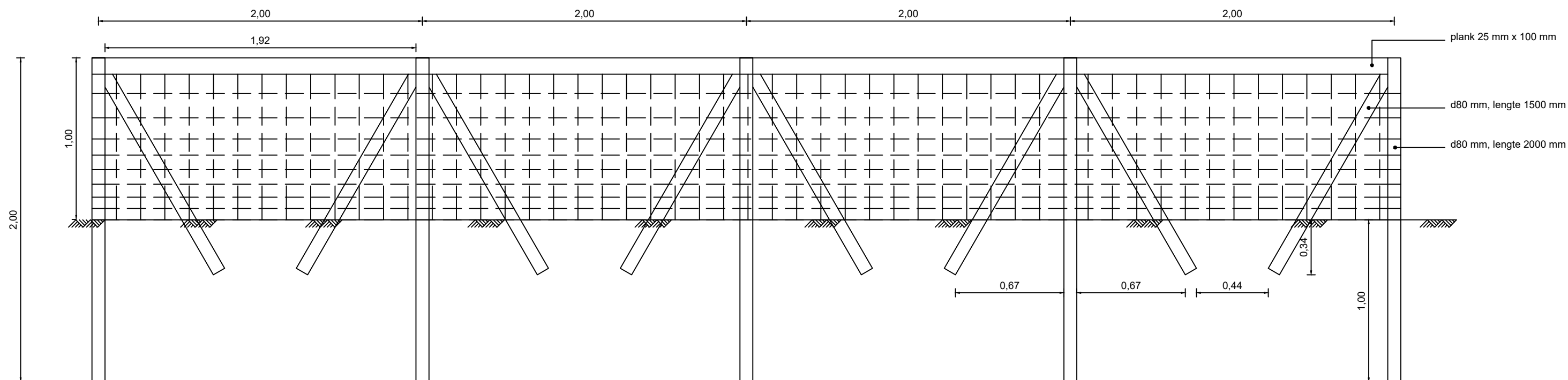
Hekwerk met schapengaas/harmonicagaas vooraanzicht Schaal 1:25
