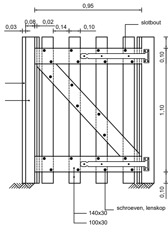
Klaphek vooraanzicht Schaal 1:20
