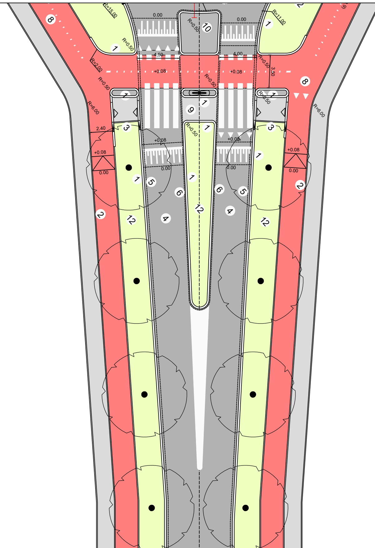
3-2-2 Gebiedsontsluitingsweg 50 km/u Schaal 1:250
