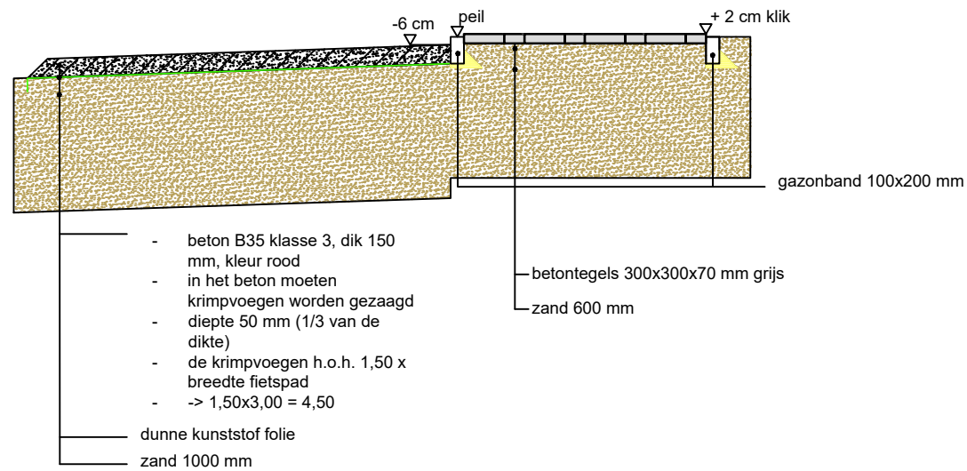
Opbouw fiets(beton)- en voet(tegel)pad Schaal 1:50
