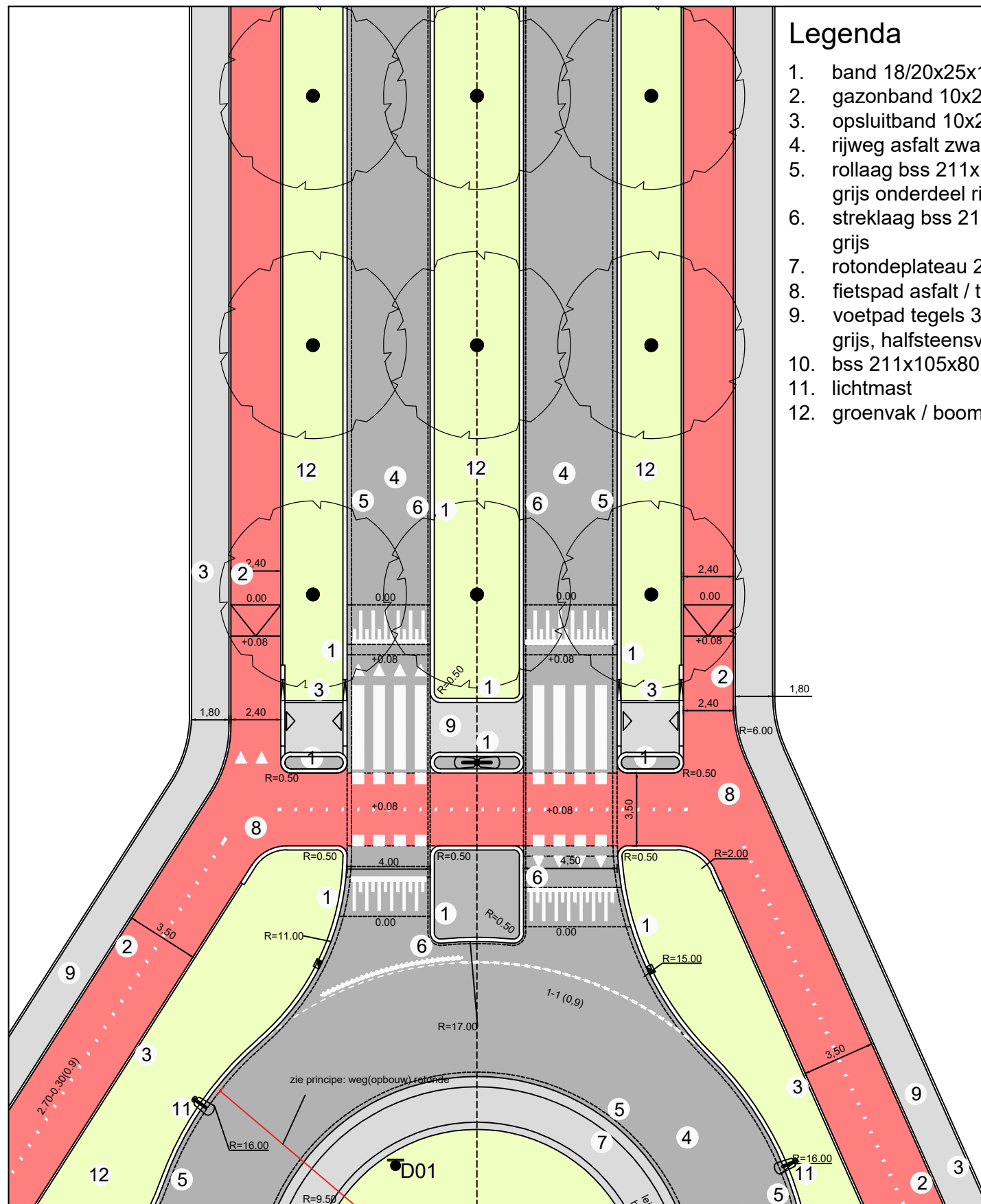
3-2-1 Hoofdweg 70 km/u Schaal 1:250
