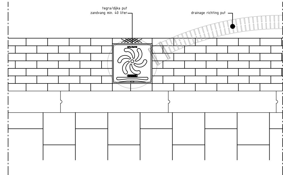
Detail waterbergende bestrating plattegrond Schaal 1:20
