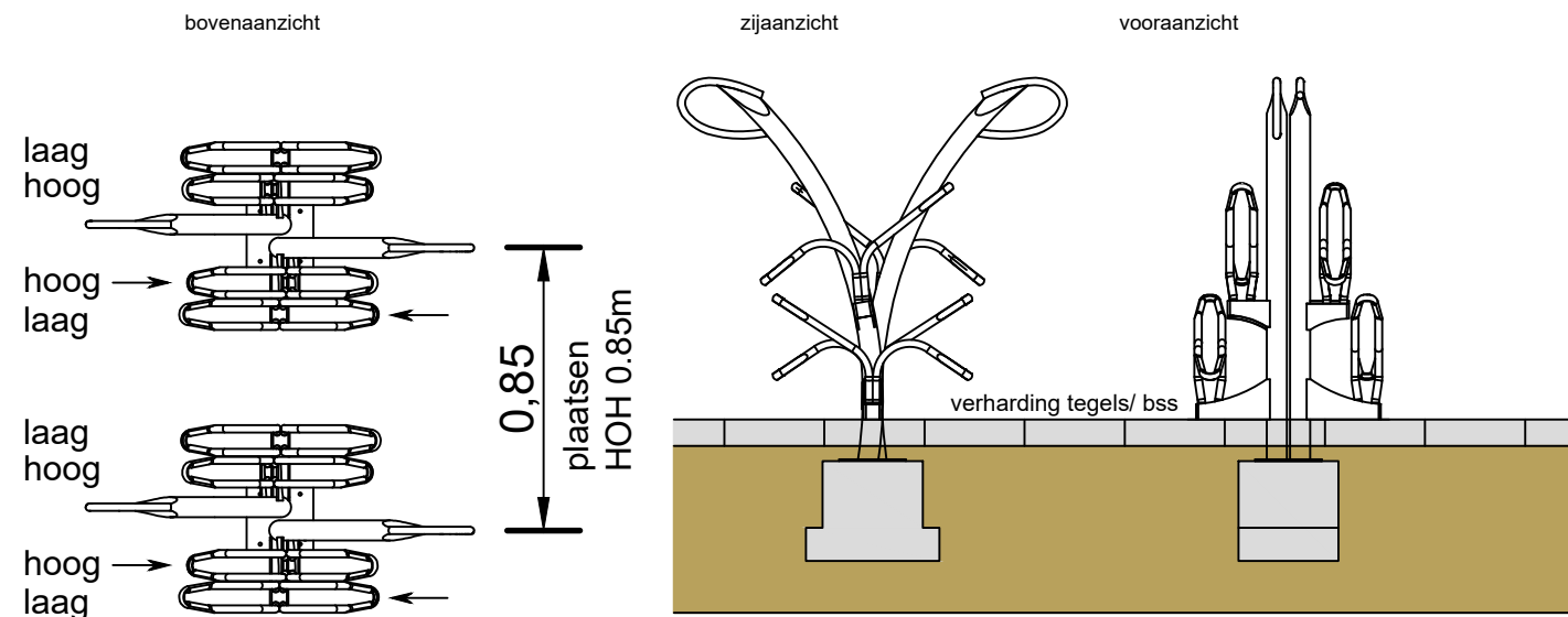
Fietsparkeren Twin Tulip
