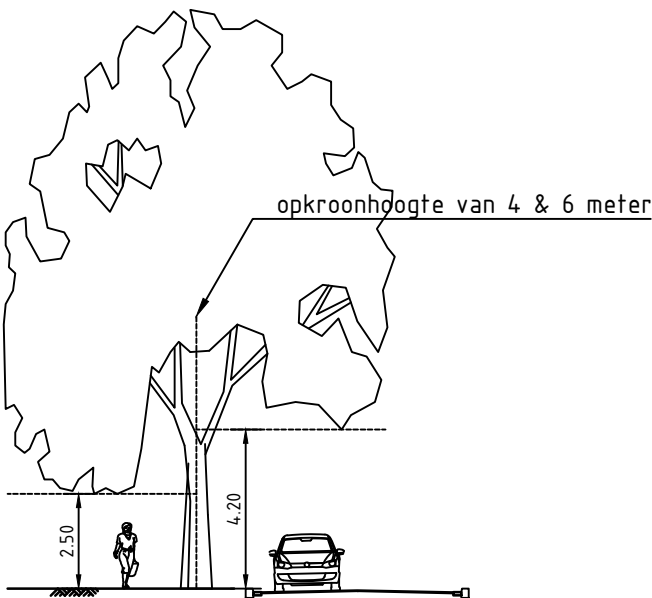
Profiel van vrije ruimte bij autoweg Schaal 1:200
