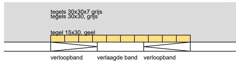
Detail D: inritconstructie Schaal 1:50
