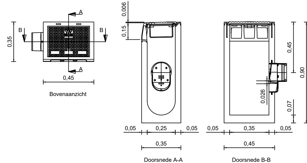
Straatkolk TRK-4717 TBS Soest Schaal 1:20
