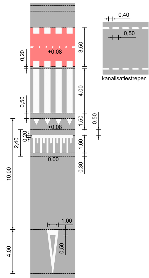
Principe: wegmarkering en belijning aanrijdroute rotonde Schaal 1:200
