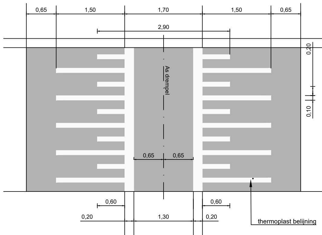
3-13-1 Asfalt sinusdrempel 50 km/u Schaal 1:50
