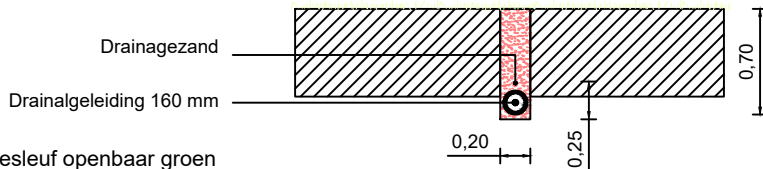
Drainagesleuf openbaar groen Schaal 1:50
