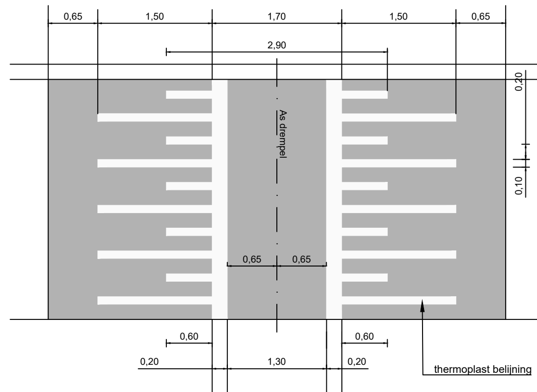
3-13-2 Asfalt sinusdrempel 50 km/u in bestaand asfalt Schaal 1:50
