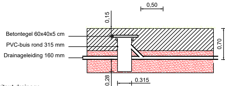
Doorspuitput drainage Schaal 1:50
