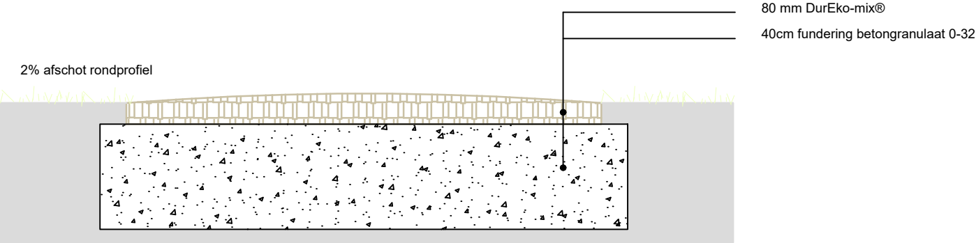
Voetpad met DurEko-mix® Schaal 1:20
