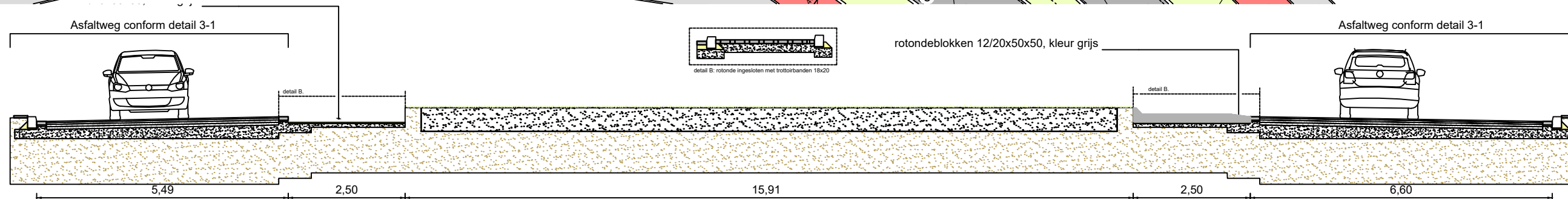
Principe: (weg)opbouw rotonde Schaal 1:100
